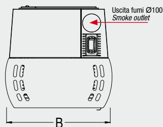
sistema di abbattimento ceneri ash collecting system
